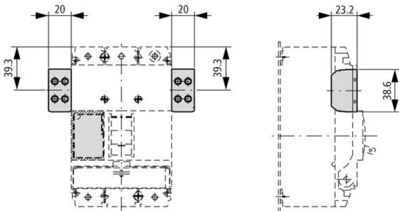
Rysunek wymiarowy: Wyzwalacz podnapięciowy do MC1, 24V DC, z kablem o dł. 3m
